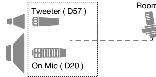
Tweeter Mix : On Mic ( D20 ) + Tweeter ( D57 )
