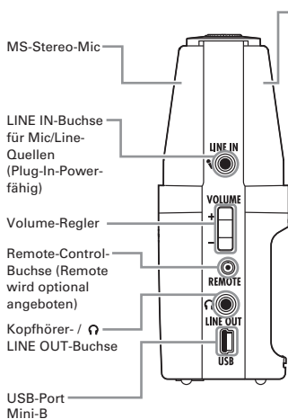
Linke Seite
